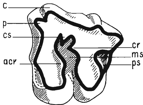
Fig. 1. — Schematyczny rysunek górnego zęba trzonowego nosorożca: acr antelidion, cr crochet, stelidion, cs crista, parastelidion, c przednie żebro, tzw. listwa, ms medisinus, główna dolina, ps postsinus, tylna dolina, p fałda parastyłu
